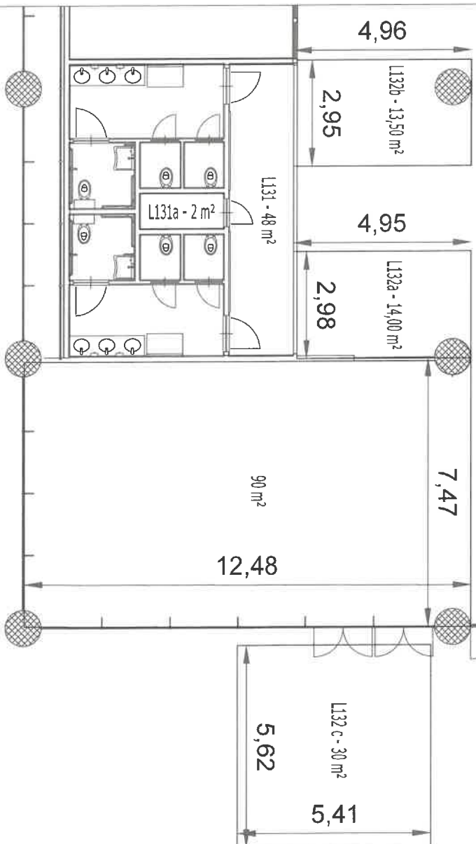
PLANIMETRIA DI DETTAGLIO SCALA 1:100
