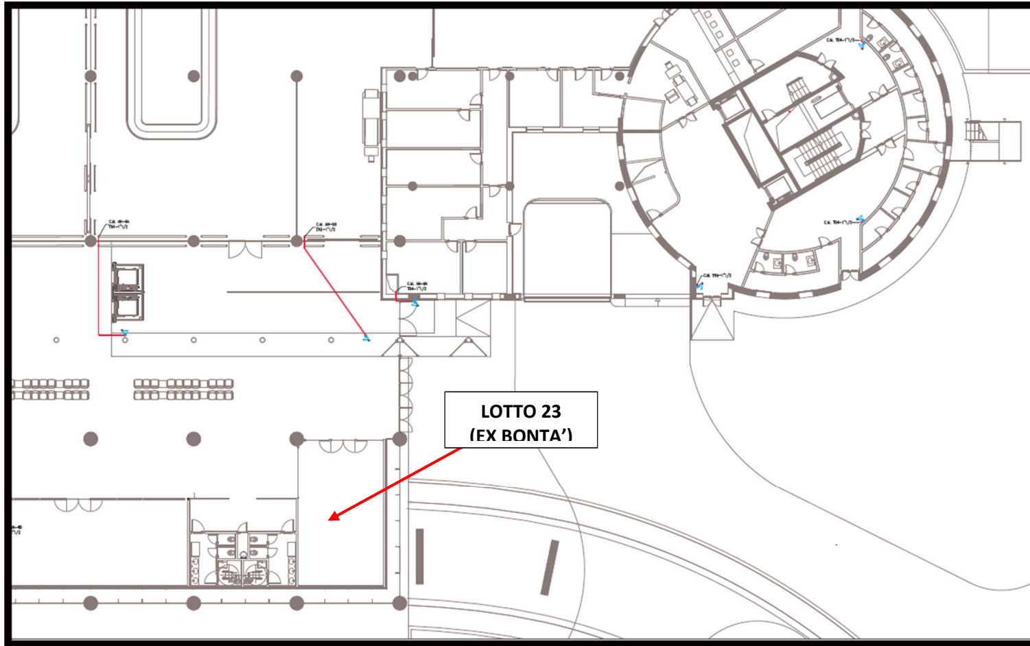
Stralcio Planimetrico terminal A – P. Terra Terminal A – RETE IDRICA ANTINCENDIO
