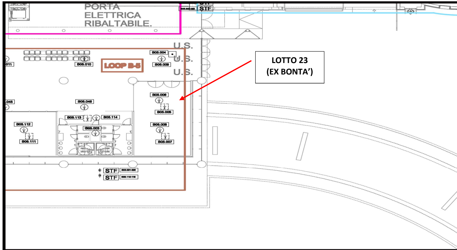
Stralcio Planimetrico terminal A – P. Terra Terminal A – LINEA LOOP E RIVELATORI FUMI
