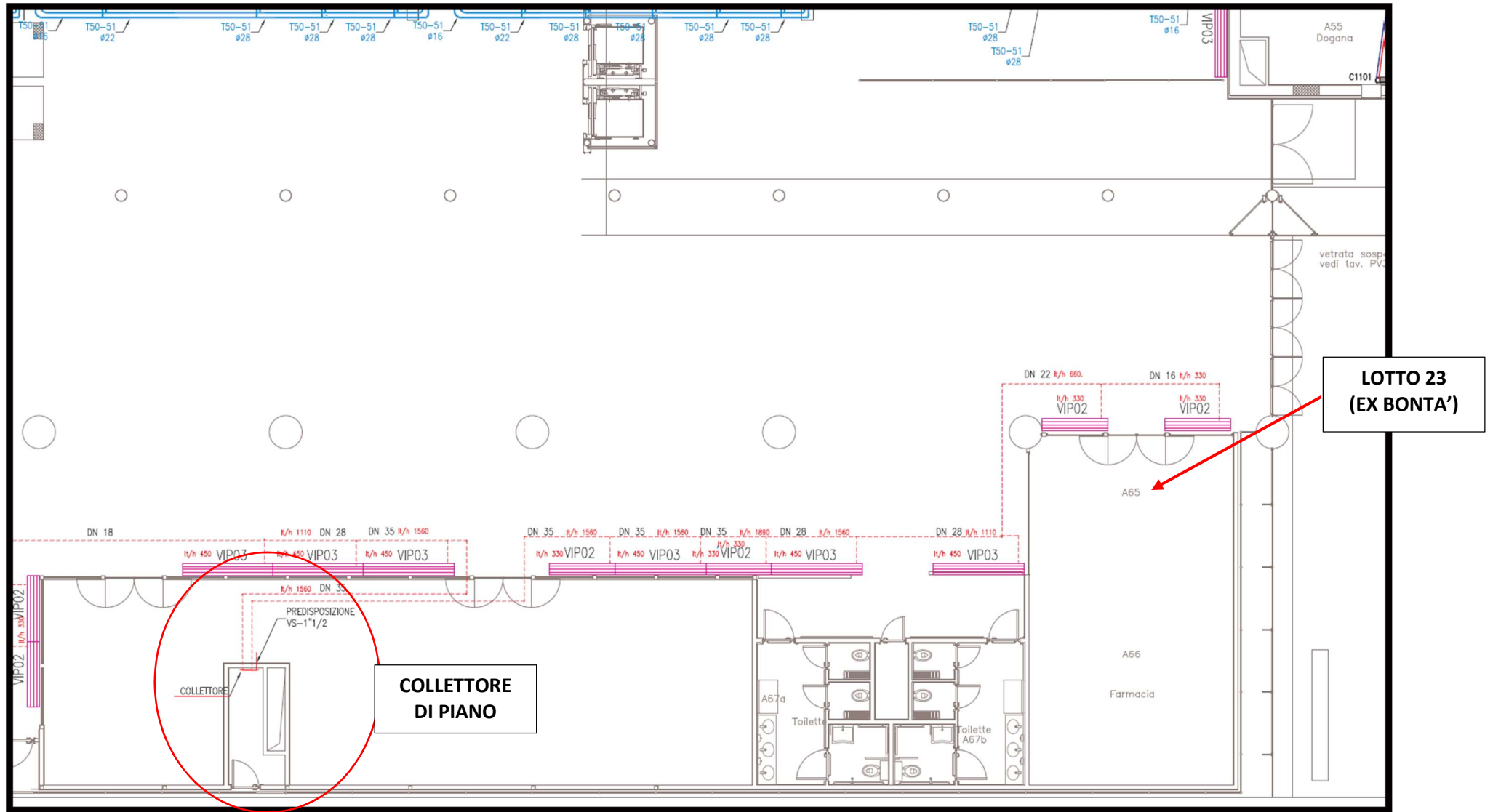
Stralcio Planimetrico terminal A – P. Terra Terminal A – LINEA CIRCUITO ACQUA REFRIGERATA FAINCOIL ( ALLA DATA DEL 2007)
