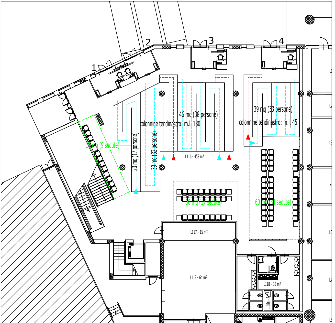
STRALCIO LIVELLO PARTENZE QUOTA + 0.00m
